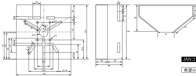
■適合する防水型カメラをポールに設置するための取付金具です。
